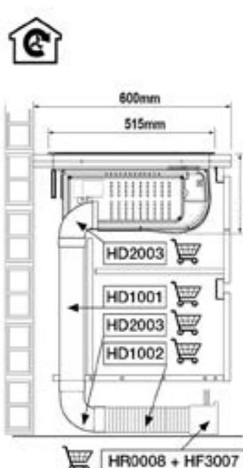
Uitvoering 1: Afvoer naar buiten
