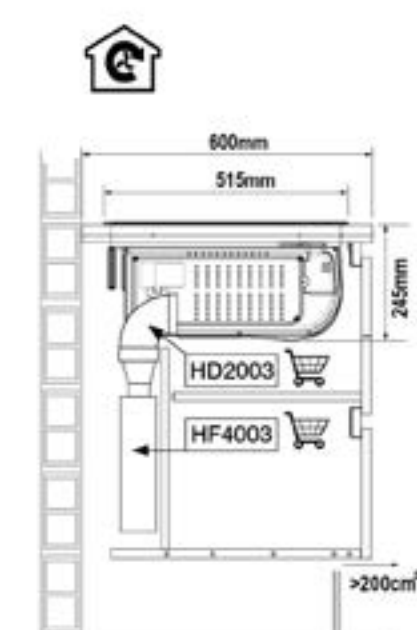
Uitvoering 2: Recirculatie met startset voor uitblaas door de achterwand
