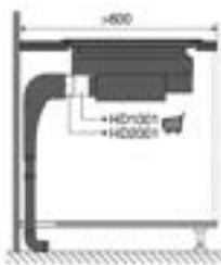
Zijaanzicht standaard afvoer en verlenging
