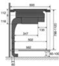
Zijaanzicht werkblad 600 mm
