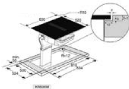
Vlak inbouw
