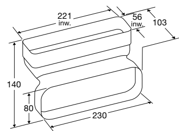
Verloopstuk bocht t.b.v. PlasmaMade filter HF4003
