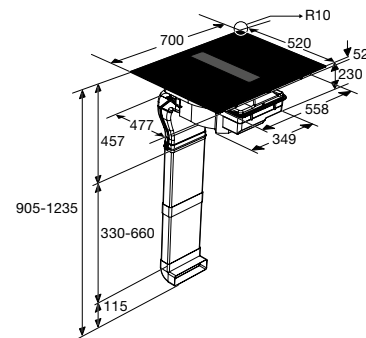
Totaal aanzicht
