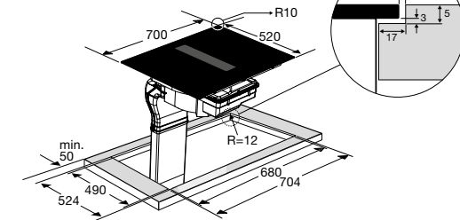
Vlak inbouw
