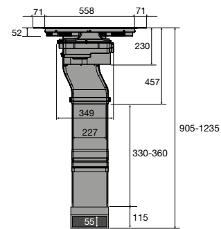
Vooraanzicht
