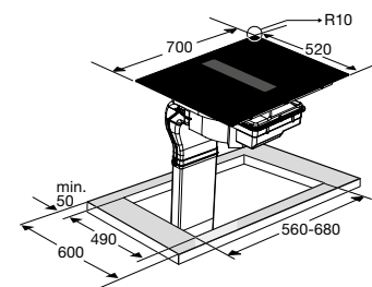
Opbouw
