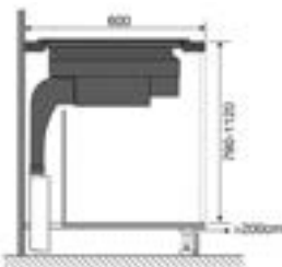
Zijaanzicht met plasmafilter
