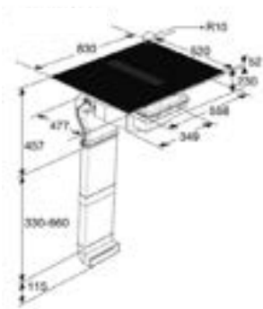
Totaal aanzicht
