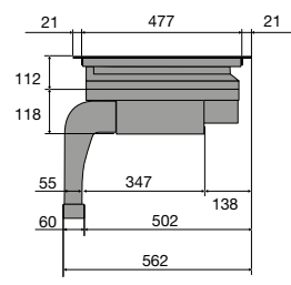
Zijaanzicht t.b.v. lade berekening
