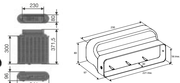
Verloopstuk recht t.b.v. PlasmaMade filter HF4003
