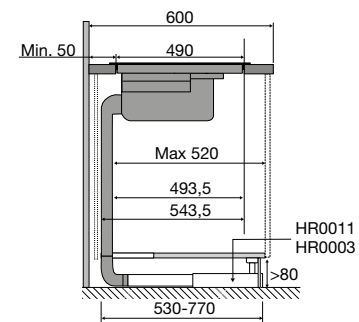
Zijaanzicht werkblad 600 mm combinatie HR0003 en HR0011
