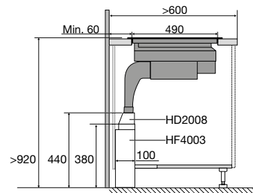
Zijaanzicht met PlasmaMade filter en adapter
