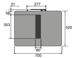
Bovenaanzicht
